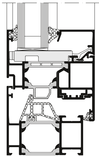
AWS 65, Escala 1:2 AWS 65, scale 1:2
